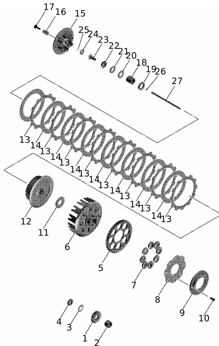
Clutch
