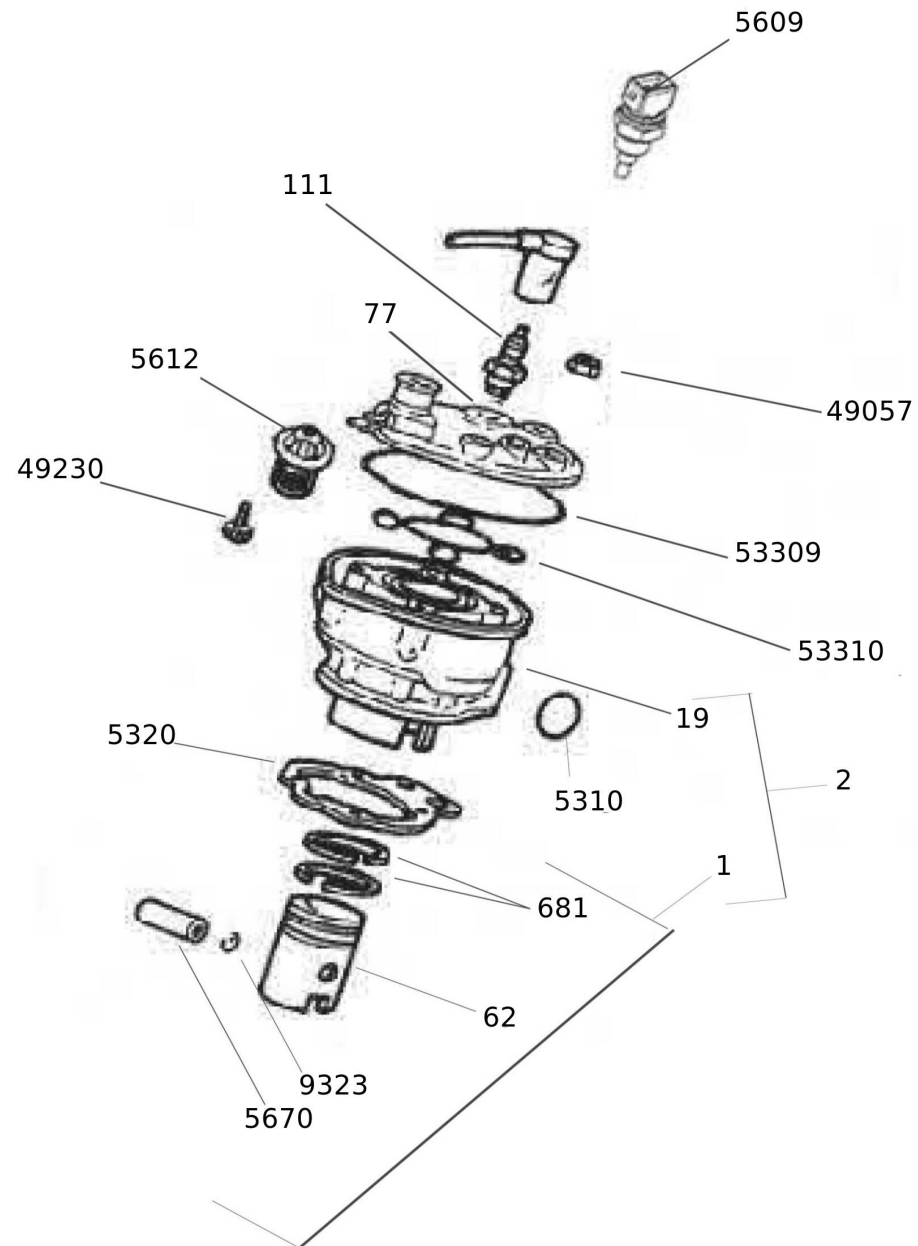
Thermal Unit
